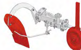
Kit aratro scalzante con / senza pulisciceppo Plant lifting plough kit with / without stump cleaner Kit charrue déchausseuse avec / sans curecep Kit arado arrancador con / sin limpiador de cepas
