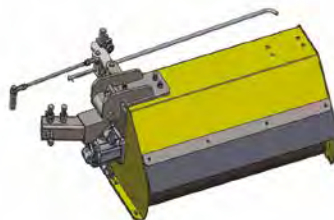
Testata mini-trincia 60/80 cm Mini-shredder head 60/80 cm Tête mini broyeur 60/80 cm Cabezal mini cosechadora 60/80 cm
