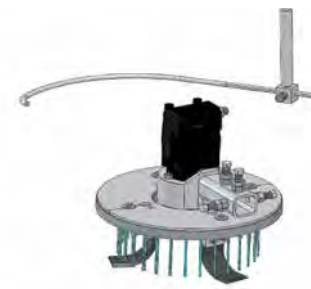
Fresino circolare 3 zappe Ø 40 cm con spazzola 3-hoes circular cutter Ø 40 cm with brush Fraise circulaire 3 houes Ø 40 cm avec brosse Fresa circular 3 azadas Ø 40 cm con escobilla
