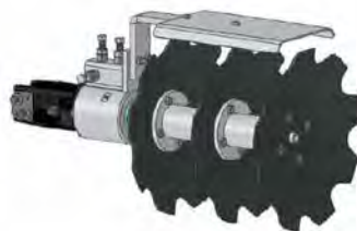
Dischiera 3 dischi rinalzanti motrici Ø 40 cm (disp. 4/5 dischi) 3 traction ridger disks kit Ø 40 cm (available 4/5 disks) Kit 3 disques à rehausser moteur Ø 40 cm (disp. 4/5 disques) Kit disco aporcador motriz a 3 discos diám. 40 cm (disp. 4/5 disco)
