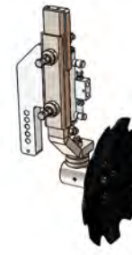
Disco rinalzante Ø 40 cm a regolazione idraulica Ridger tiller disc Ø 40 cm with hydraulic adjustment Disque rehausseur Ø 40 à réglage hydraulique Disco aporcador Ø 40 con carrera hidráulico
