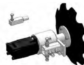
Fresino circolare 3 zappe Ø 40 cm con spazzola 3-hoes circular cutter Ø 40 cm with brush Fraise circulaire 3 houes Ø 40 cm avec brosse Fresa circular 3 azadas Ø 40 cm con escobilla
