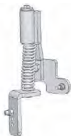
Ammortizzatore paraterra orientabile e rinforzato Adjustable and reinforced shock absorber Amortisseur defense terre réglable et renforcé Amortiguador paratierra regulable y reforzado
