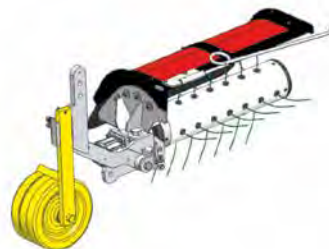
Trinciaerba a fili verticali Vertical wires mower Hache-herbe a fils verticaux Picadora de hierba de hilos verticales
