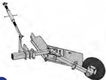
Paraterra per Frutteto (anche con disco delimitatore) Ground cover for Orchard (also with delimeter disc) Défense terre pour Arboricole (aussi avec disk delimiteur) Paratierra para Frutales (también con disco delimitator)
