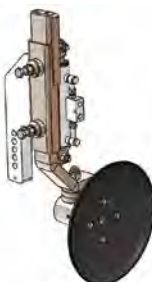
Disco apripista bombato Ø 36 cm a regolazione idraulica Rounded tiller disc Ø 36 cm with hydraulic adjustment Disque boteur bombé Ø 36 cm avec course hydraulique Disco de empuje abombado con carrera hidráulico
